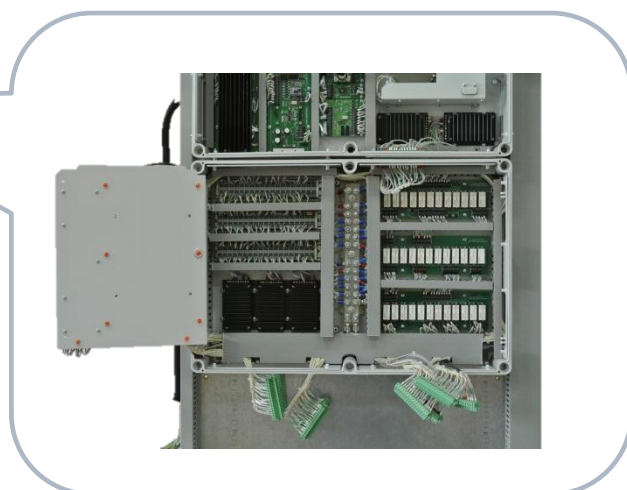
Стойка электрооборудования ЭО
