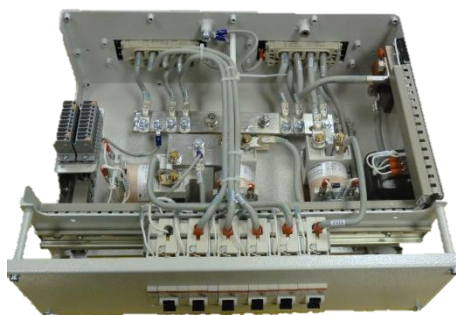
Модуль блока распределительного БР
